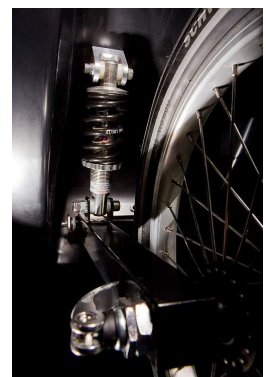
Ein einstellbares Federbein sorgt für Komfort.
